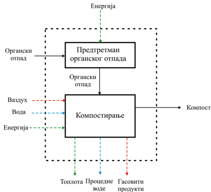
Слика 2.7 Блок шема токова отпада и емисија приликом компостирања
