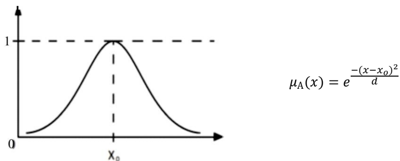
Слика 5.15 Гаусова функција припадности
