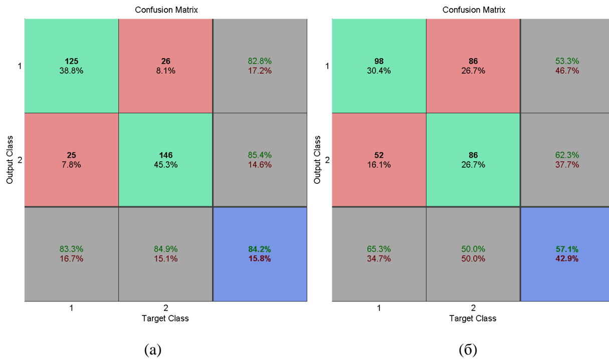
SVM класификација;
