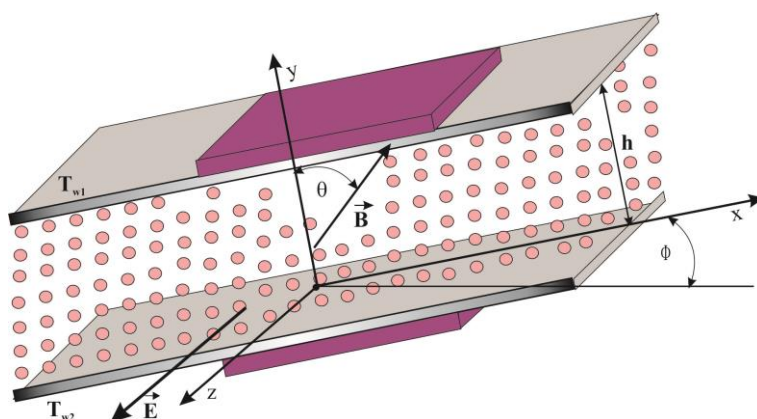
Slika 5a Fizički model strujanja
