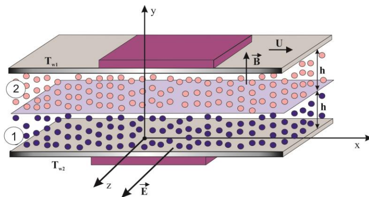
Slika 4b Fizički model strujanja
