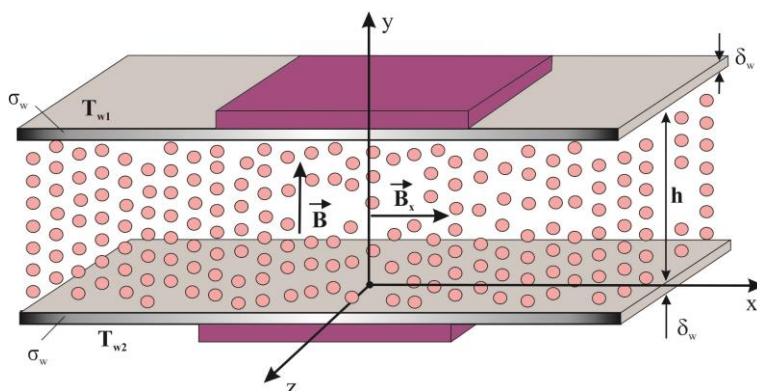
Slika 3e Fizički model strujanja
