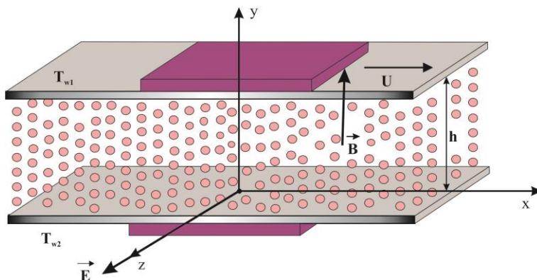
Slika 3b Fizički model strujanja
