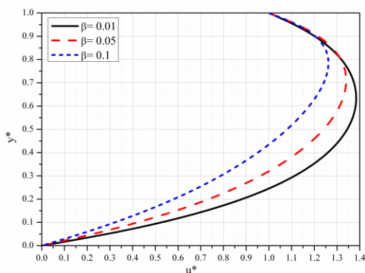
Slika 5.27 Bezdimeziono uzdužna brzina za različite vrednosti parametra \beta
