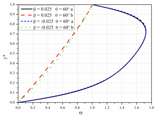
Slika 5.64 Bezdimezijska temperatura za različite vrednosti \beta i \theta = 60^\circ
