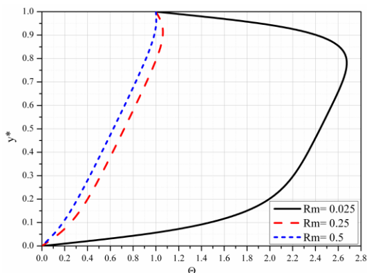
Slika 5.43 Bezdimeziona temperatura za različite vrednosti R_m
