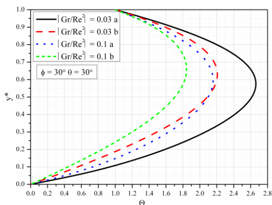
Slika 5.76 Bezdimezijska temperatura za različite vrijednosti Gr/Re^2 , \phi = 30^\circ , \theta = 30^\circ
