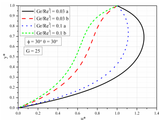
Slika 5.75 Bezdimezijska brzina za različite vrijednosti Gr/Re^2 , \phi = 30^\circ , \theta = 30^\circ
