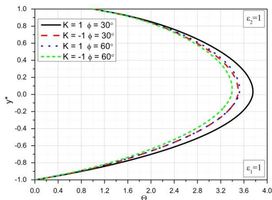
Slika 6.6 Bezdimezijska temperatura za različite vrednosti K i \phi
