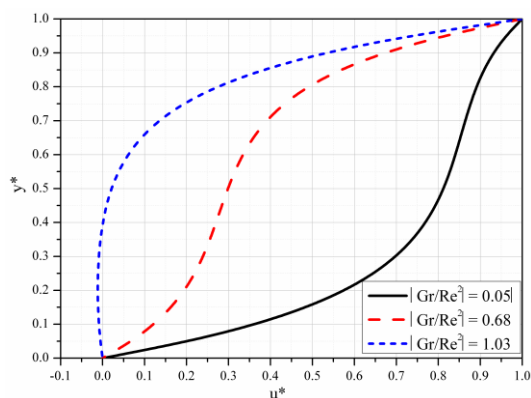
Slika 5.25 Bezdimeziona uzdužna brzina za različite vrednosti Gr/Re^2
