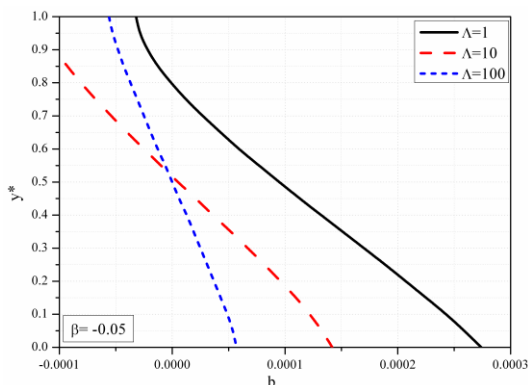
Slika 3.48b Bezdimeziona indukcija za različite vrednosti \Lambda , \beta = -0.05 , c = 1
