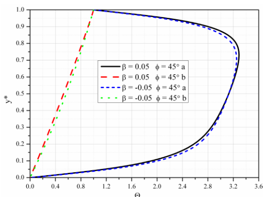
Slika 5.53 Bezdimeziono temperatura za različite vrednosti \beta i \phi = 45^\circ
