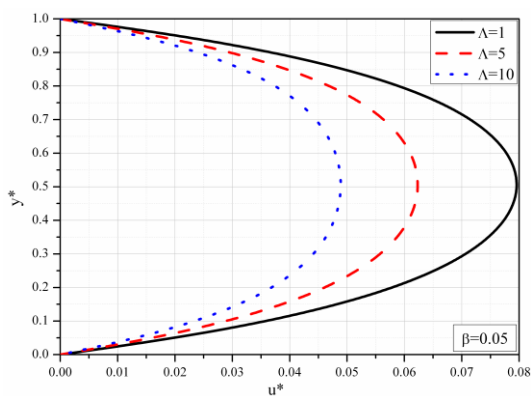
Slika 3.18 Bezdimezionna uzdužna brzina za različite vrednosti \Lambda
