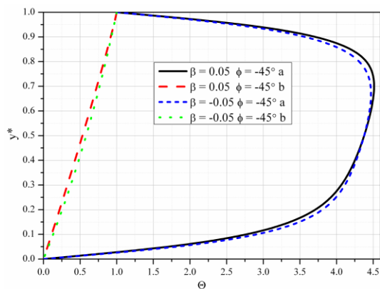
Slika 5.54 Bezdimenziona temperatura za različite vrednosti \beta i \phi = -45^\circ
