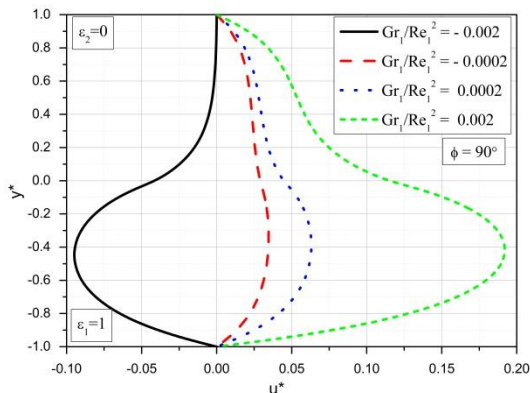
Slika 6.25 Bezdimezionna uzdužna brzina
