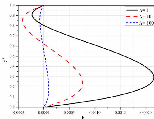
Slika 5.39 Bezdimezijska magnetna indukcija za različite vrednosti \Lambda
