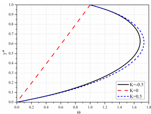
Slika 5.6 Bezdimezijska temperatura za različite vrednosti K
