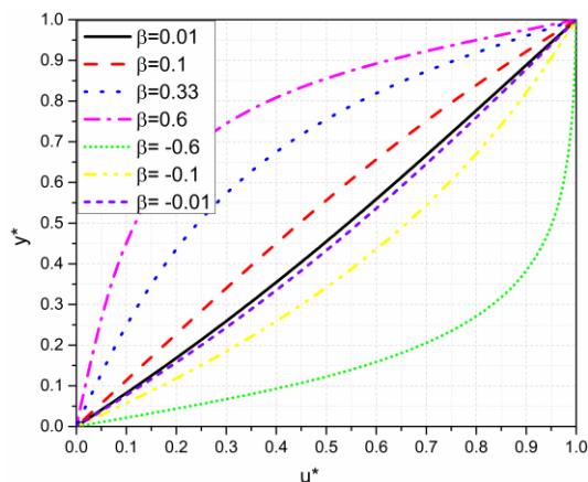
Slika 3.10 Raspored bezdimenzione brzine za različite vrednosti \beta
