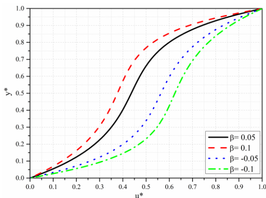
Slika 3.32 Bezdimezijska uzdužna brzina za različite vrednosti \beta
