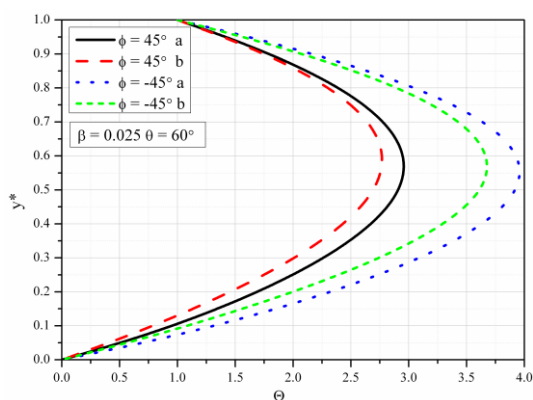
Slika 5.78 Bezdimezijska temperatura za različite vrednosti \phi
