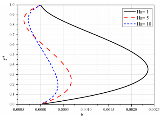
Slika 5.36 Bezdimezijska magnetna indukcija za različite vrednosti Ha
