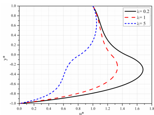
Slika 4.13 Bezdimenziona brzina za različite vrednosti parametra \lambda
