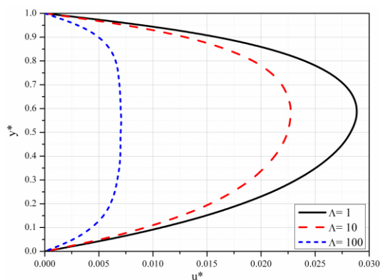
Slika 5.3 Raspored bezdimenzionirane uzdužne brzine za različite vrednosti faktora poroznosti
