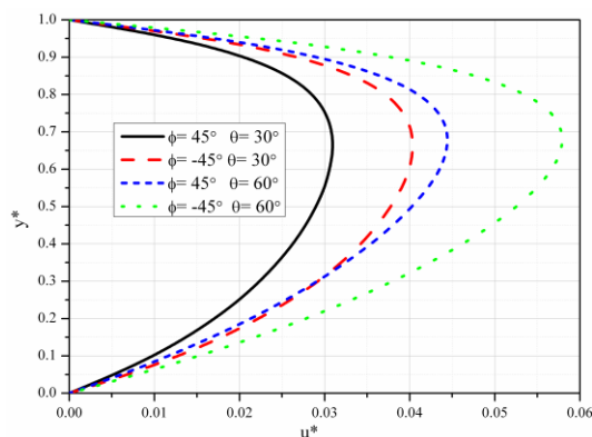
Slika 5.15 Bezdimezijska uzdužna brzina za različite vrednosti \phi i \theta
