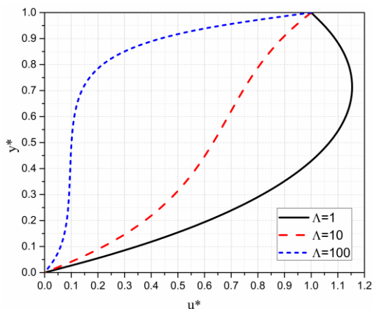
Slika 3.11 Raspojed bezdimenzionih brzina za različite vrijednosti \Lambda
