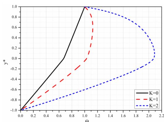
Slika 4.12 Bezdimezijska temperatura za različite vrednosti K
