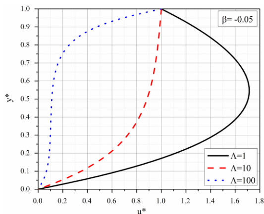
Slika 3.29b Bezdimeziorna uzdužna brzina za različite vrednosti \Lambda ; \beta = -0.05
