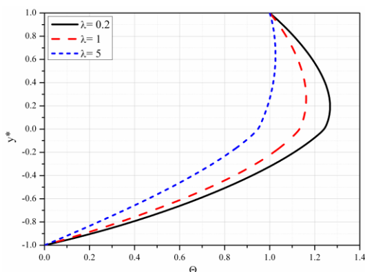
Slika 4.2 Bezdimezijska temperatura za različite vrednosti odnosa parametara poroznosti \lambda
