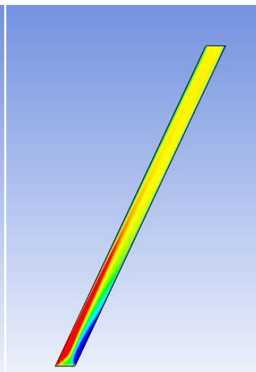
Slika 7.37 Polje brzine Ha = 25
