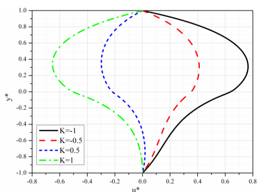
Slika 4.11 Bezdimezijska brzina za različite vrednosti K
