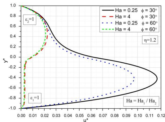
Slika 6.3 Bezdimezionna uzdužna brzina za različite vrednosti Ha i \phi
