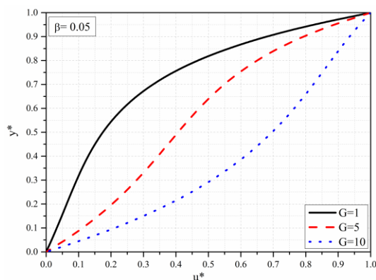
Slika 3.31a Bezdimezionirana uzdužna brzina za različite vrednosti G , \beta = 0.05
