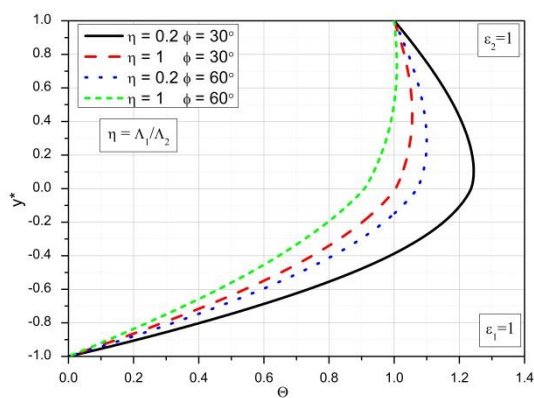
Slika 6.2 Bezdimezionna temperatura za različite vrednosti \eta i \phi
