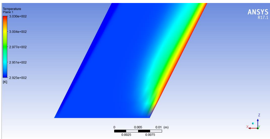
Slika 7.34 Polje temperature u kosom kanalu
