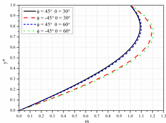
Slika 5.32 Bezdimezijska temperatura za različite vrednosti \phi i \theta
