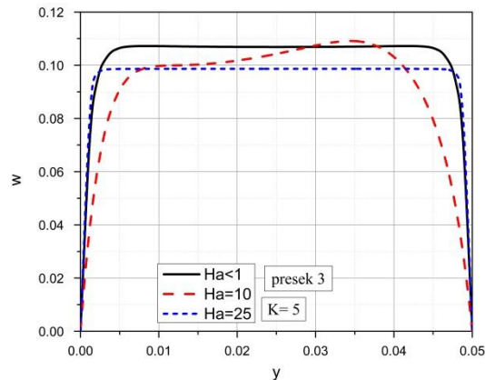
Slika 7.30 Uticaj Hartmann-ovog broja na komponentu brzine u z pravcu
