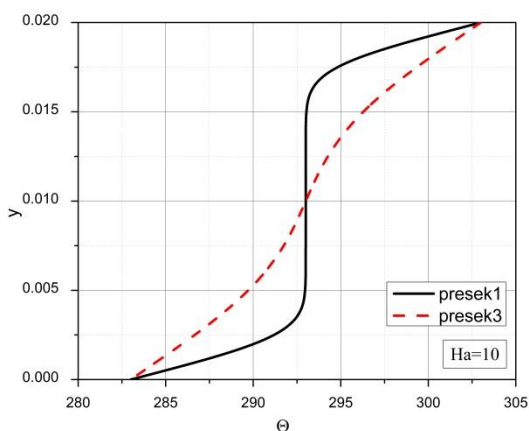
Slika 7.13 Temperatura u različitim preseccima kanala
