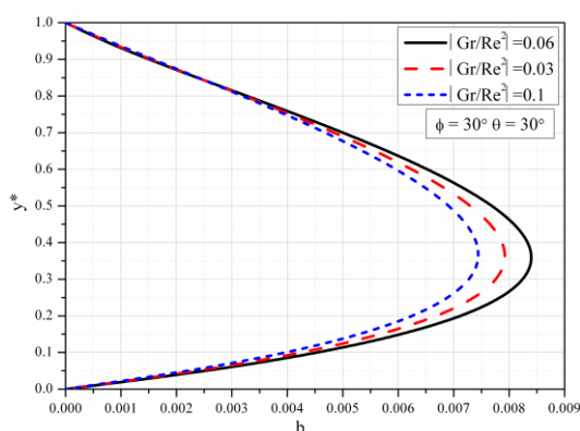
Slika 5.74 Bezdimezionno magnetno polje za različite vrednosti Gr/Re^2 , \phi = 30^\circ , \theta = 30^\circ
