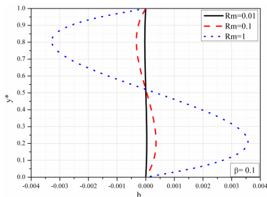
Slika 3.23 Bezdimezijska indukcija indukovano magnetnog polja za različite vrednosti R_m
