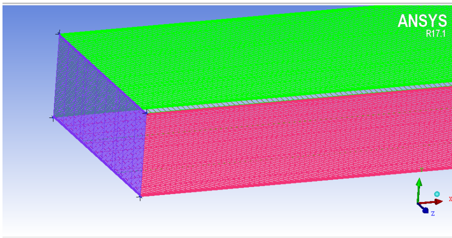
Slika 7.3 Detalj domena strujanja
