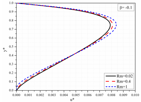
Slika 3.46b Bezdimezijska uzdužna brzina za različite vrednosti R_m , \beta = -0.1, c = 1, Ha = 10
