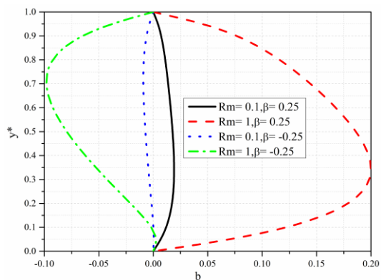
Slika 3.38 Bezdimeziona indukcija indukovanog magnetnog polja za razliĉite vrednosti Rm i \beta
