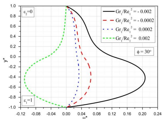
Slika 6.23 Bezdimezionna uzdužna brzina za različite vrednosti Gr_1/Re_1^2 i \phi = 30^\circ
