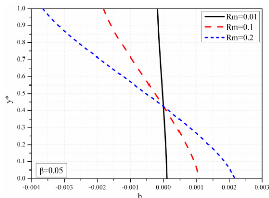
Slika 3.49a Bezdimezijska indukcija za različite vrednosti R_m , \beta = 0.05 , c = 1
