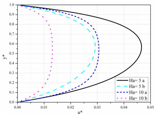
Slika 5.35 Bezdimezijska uzdužna brzina za različite vrednosti Ha
