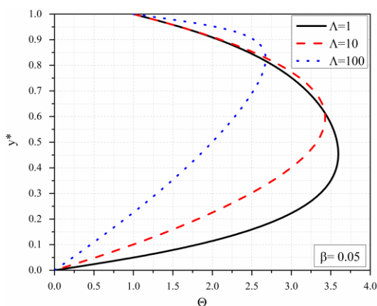
Slika 3.39a Bezdimeziona temperatura za različite vrednosti \Lambda , \beta = 0.05
