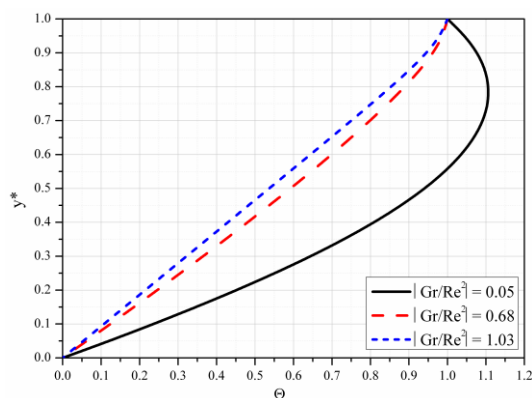
Slika 5.26 Bezdimeziona temperatura za različite vrednosti Gr/Re^2
