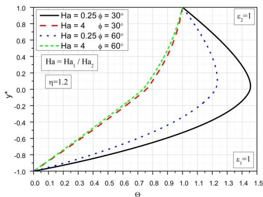
Slika 6.4 Bezdimezionna temperatura za različite vrednosti Ha i \phi
