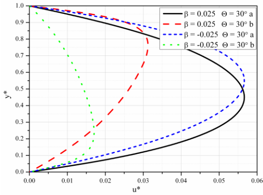
Slika 5.60 Bezdimezijska uzdužna brzina za različite vrednosti \beta i \theta = 30^\circ
