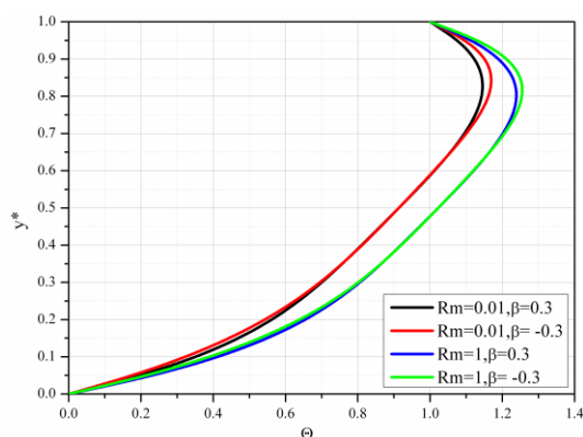
Slika 3.27 Bezdimezionona temperatura za različite vrednosti Rm i \beta
