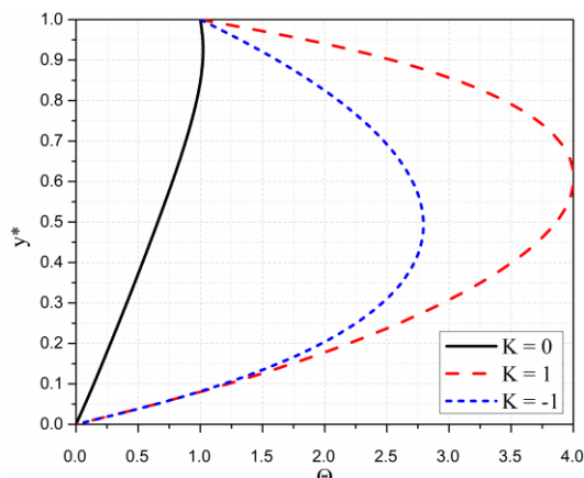
Slika 3.16 Raspori bezdimenzionih temperatura za različite vrednosti K
