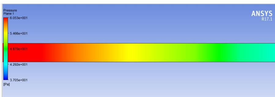
Slika 7. 17 Polje pritiska u kanalu
