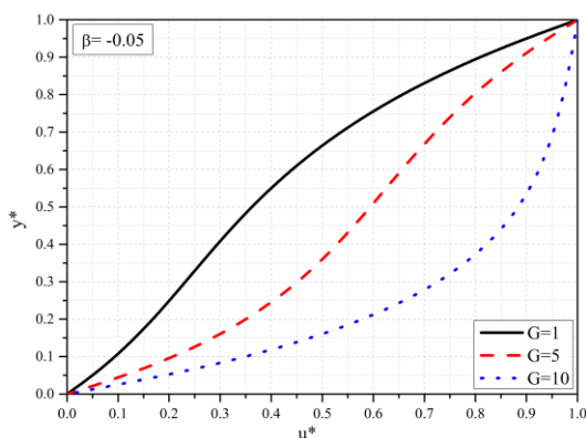
Slika 3.31b Bezdimezionirana uzdužna brzina za različite vrednosti G , \beta = -0.05
