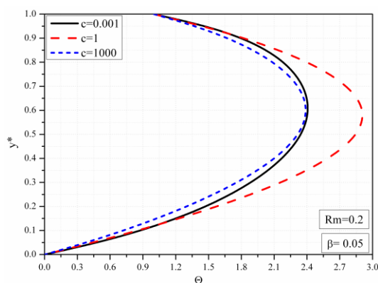
Slika 3.54 Bezdimeziona temperatura za različite vrednosti c , \beta = 0.05
