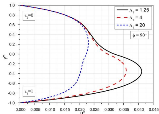
Slika 6.13 Bezdimezijska uzdužna brzina za različite vrednosti \Lambda_1 i \phi = 90^\circ
