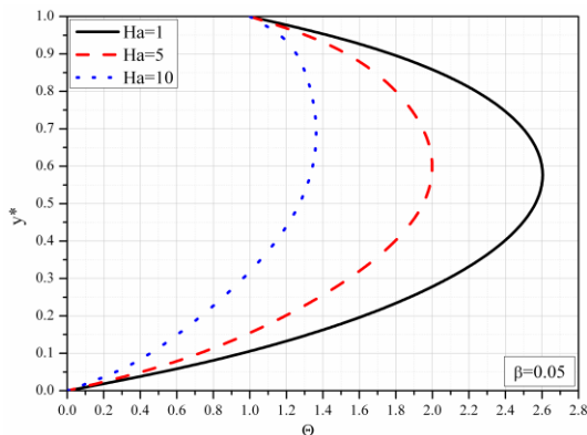
Slika 3.25 Bezdimezijska temperatura za različite vrednosti Ha
