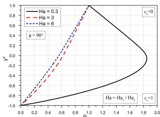
Slika 6.18 Bezdimeziona temperatura za različite vrednosti Ha i \phi = 90^\circ
