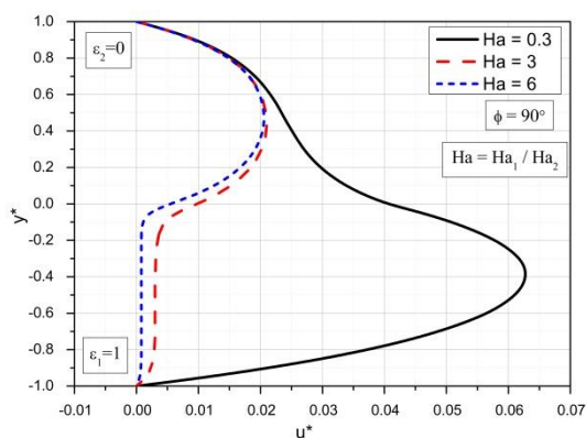
Slika 6.17 Bezdimeziona uzdužna brzina za različite vrednosti Ha i \phi = 90^\circ
