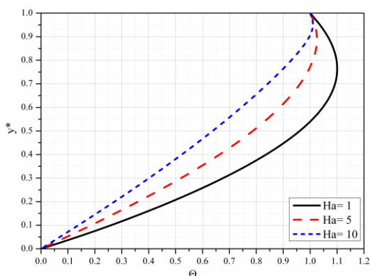
Slika 5.20 Bezdimeziono temperatura za različite vrednosti Ha
