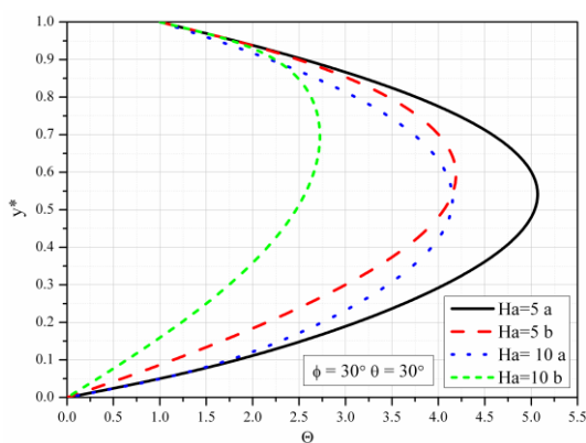
Slika 5.67 Bezdimezionna temperatura za različite vrednosti Ha broja, \phi = 30^\circ , \theta = 30^\circ
