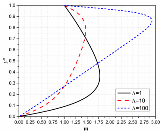
Slika 3.15 Raspori bezdimenzionih temperatura za različite vrednosti \Lambda
