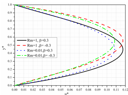
Slika 3.19 Bezdimeziona uzdužna brzina za različite vrednosti Rm i \beta
