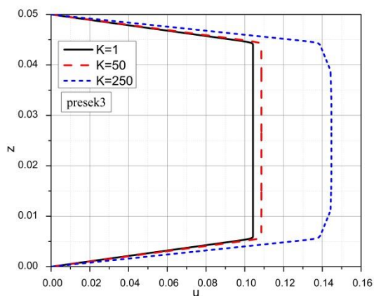
Slika 7.10 Bezdimezijska uzdužna brzina za različite vrednosti faktora otpora sredine
