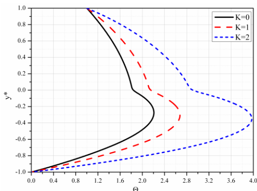
Slika 4.18 Bezdimezijska temperatura za različite vrednosti K
