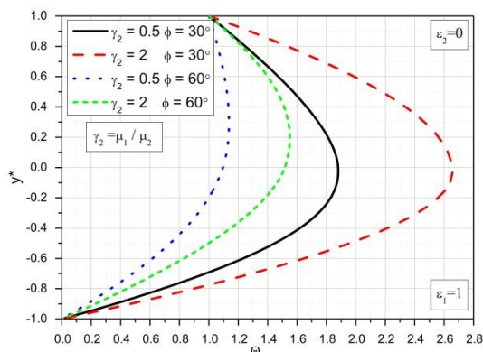
Slika 6.20 Bezdimezijska temperatura za različite vrednosti \gamma_2 i \phi
