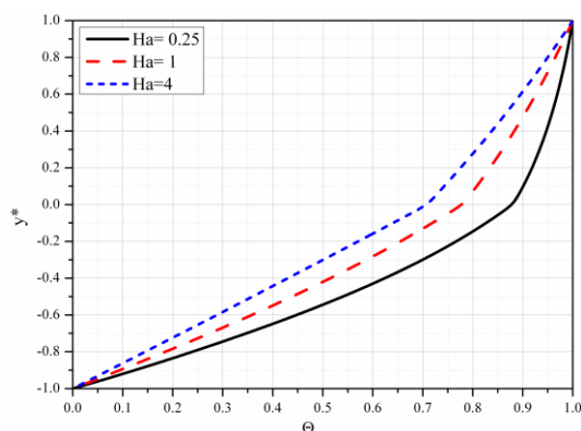
Slika 4.4 Bezdimezijska temperatura za različite vrednosti Ha
