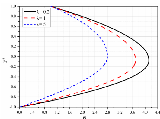
Slika 4.14 Bezdimenziona temperatura za različite vrednosti parametra \lambda
