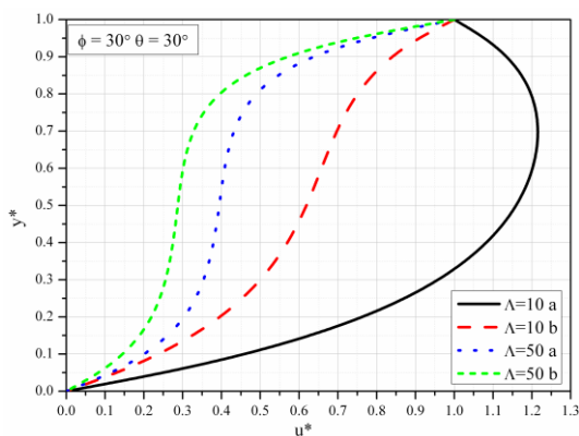
Slika 5.69 Bezdimeziona brzina za različite vrednosti \Lambda , \phi = 30^\circ , \theta = 30^\circ
