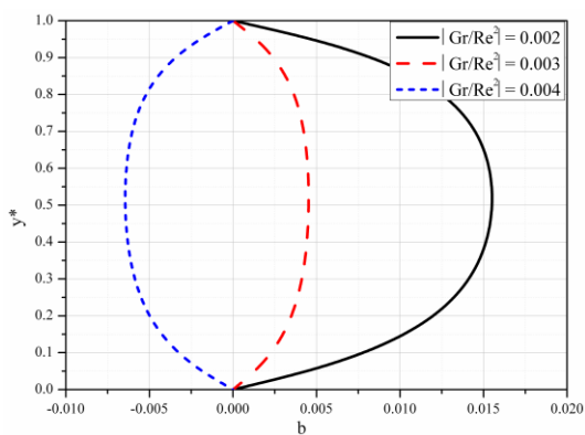
Slika 5.48 Bezdimeziona magnetna indukcija za različite vrednosti Gr/Re^2
