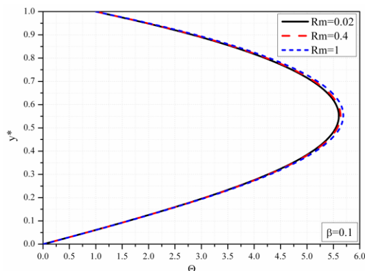
Slika 3.52a Bezdimezijska temperatura za različite vrednosti Rm , \beta = 0.1 , c = 1
