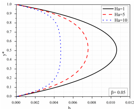
Slika 3.35 Bezdimeziiona indukcija indukovanog magnetnog polja za različite vrednosti Ha , \beta = 0,05
