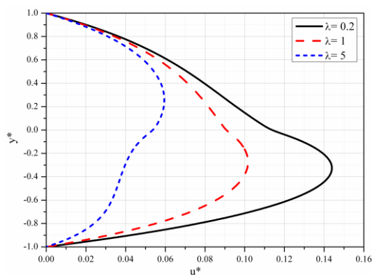
Slika 4.1 Bezdimezijska brzina za različite vrednosti odnosa parametara poroznosti \lambda
