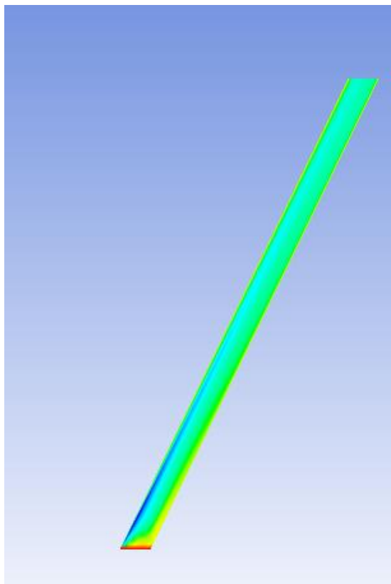
Slika 7.31 Komponenta brzine u u kosom kanalu
