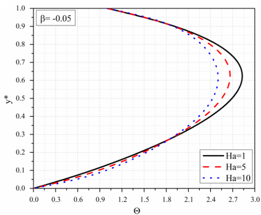
Slika 3.40b Bezdimeziona temperatura za različite vrednosti Ha , \beta = -0.05
