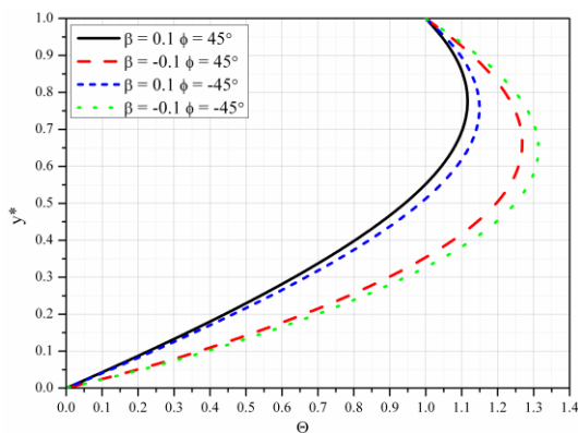
Slika 5.30 Bezdimezijska temperatura za različite vrednosti \beta i \phi
