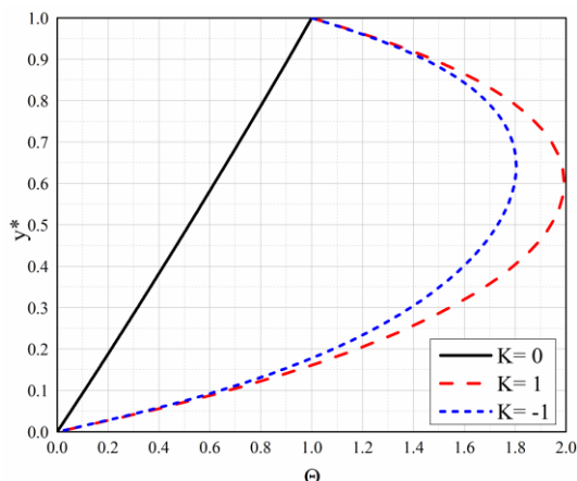
Slika 3.8 Rasped bezdimenzionane temperature za različite vrednosti faktora električnog opterećenja
