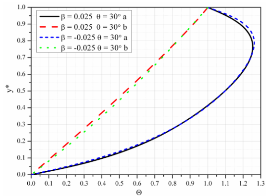
Slika 5.63 Bezdimezijska temperatura za različite vrednosti \beta i \theta = 30^\circ
