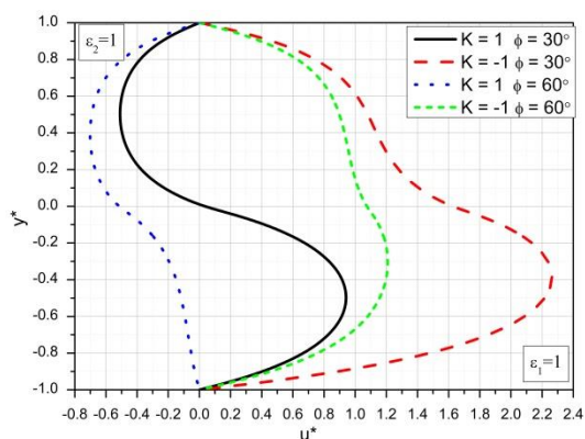
Slika 6.5 Bezdimezijska uzduzna brzina za različite vrednosti K i \phi
