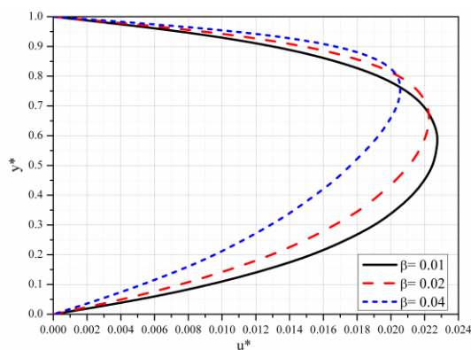
Slika 5.11 Bezdimeziona uzdužna brzina za različite vrednosti \beta
