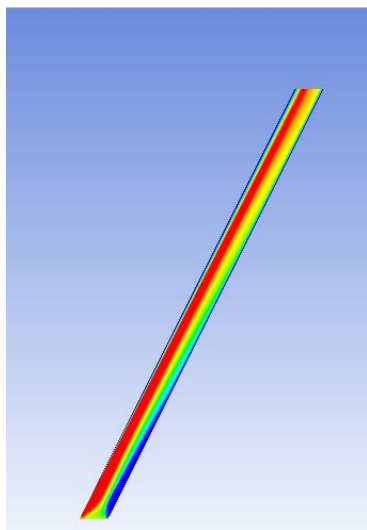
Slika 7.35 Polje brzine Ha < 1
