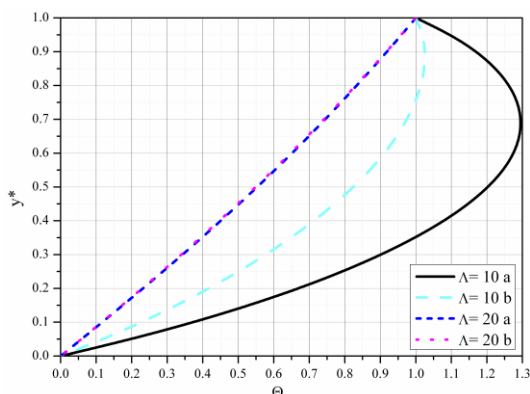
Slika 5.40 Bezdimezijska temperatura za različite vrednosti \Lambda
