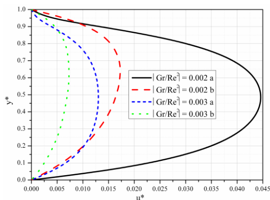
Slika 5.47 Bezdimeziona uzdužna brzina za različite vrednosti Gr/Re^2
