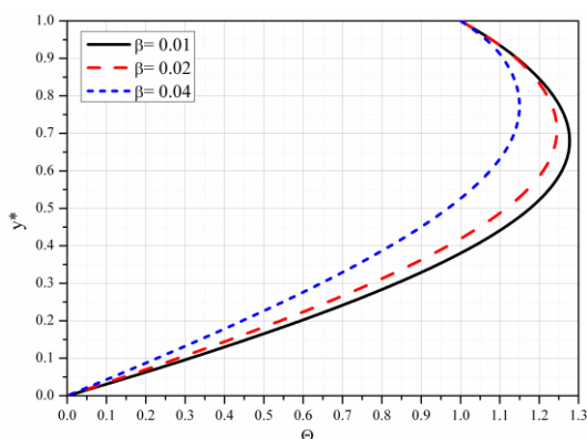
Slika 5.12 Bezdimeziona temperatura za različite vrednosti \beta
