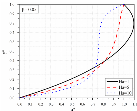
Slika 3.30a Bezdimezijska uzduzna brzina za različite vrednosti Ha , \beta = 0.05
