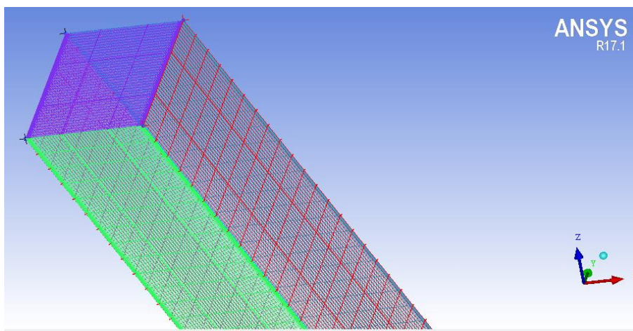
Slika 7.20 Detalj domena strujanja u kosom kanalu
