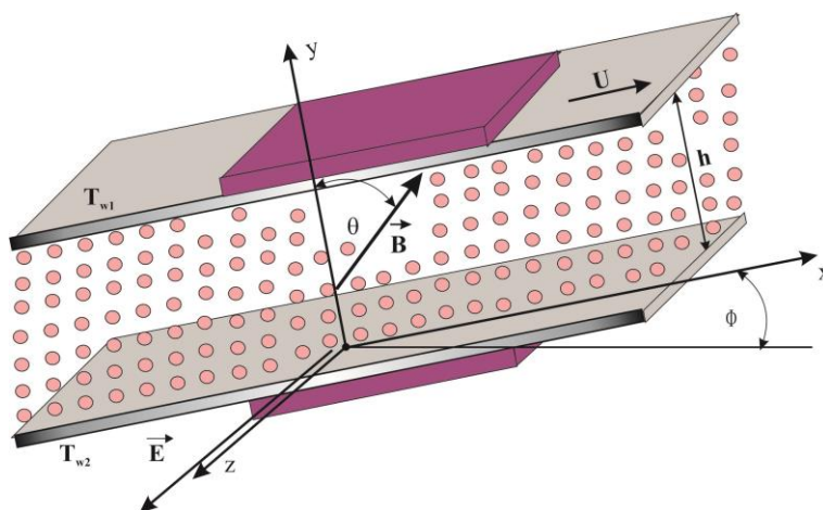
Slika 5b Fizički model strujanja
