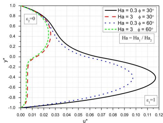
Slika 6.15 Bezdimezijska uzdužna brzina za različite vrednosti Ha i \phi
