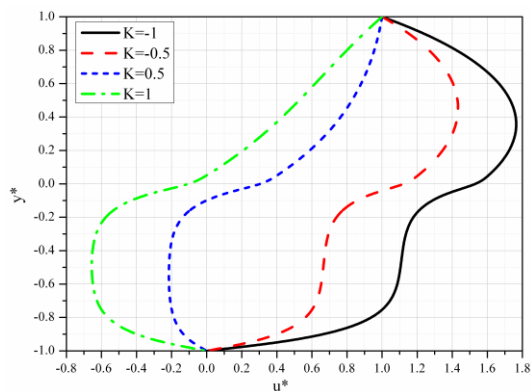
Slika 4.23 Bezdimenziona brzina za različite vrednosti K
