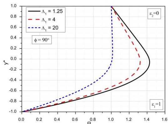
Slika 6.14 Bezdimezijska temperatura za različite vrednosti \Lambda_1 i \phi = 90^\circ
