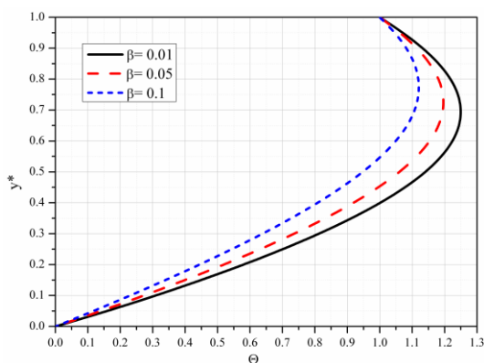
Slika 5.28 Bezdimeziono temperatura za različite vrednosti parametra \beta
