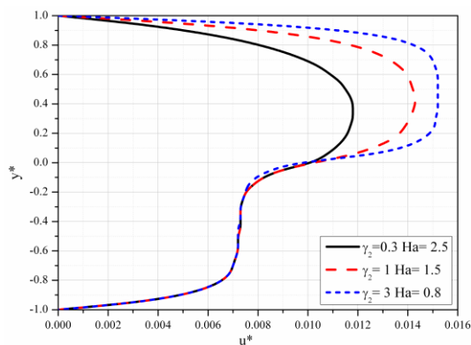
Slika 4.7 Bezdimezijska brzina za različite vrednosti odnosa viskoznosti \gamma_2
