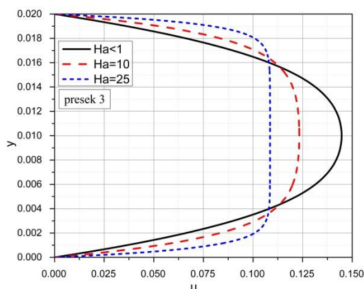
Slika 7.11 Bezdimezijska uzdužna brzina za različite vrednosti Hartmann-ovog broja
