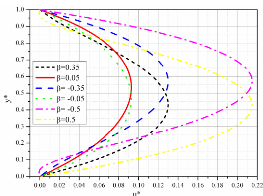
Slika 3.20 Bezdimeziona uzdužna brzina za različite vrednosti \beta
