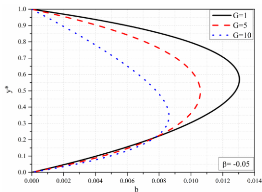
Slika 3.36b Bezdimeziona indukcija indukovanog magnetnog polja za razliĉite vrednosti G , \beta = -0.05
