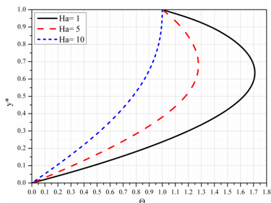
Slika 5.2 Rasplet bezdimenzionirane temperature za različite vrednosti Hartmann-ovog broja
