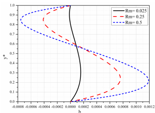
Slika 5.42 Bezdimeziona magnetna indukcija za različite vrednosti Rm
