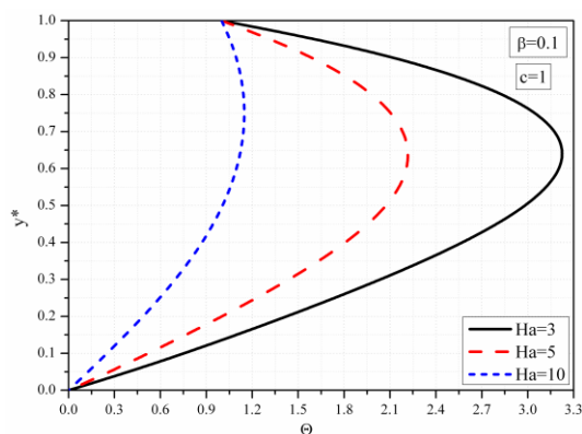
Slika 3.50a Bezdimezionna temperatura za različite vrednosti Ha , \beta = 0.1
