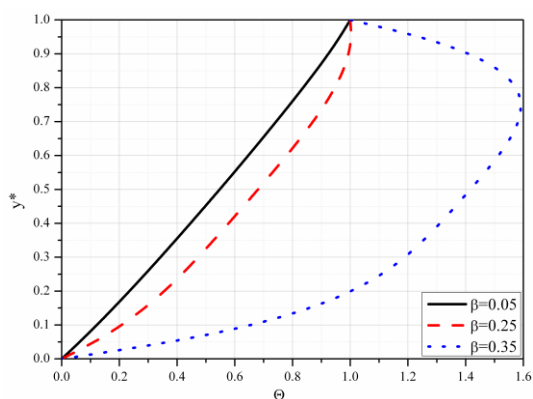
Slika 3.28 Bezdimezionona temperatura za različite vrednosti \beta
