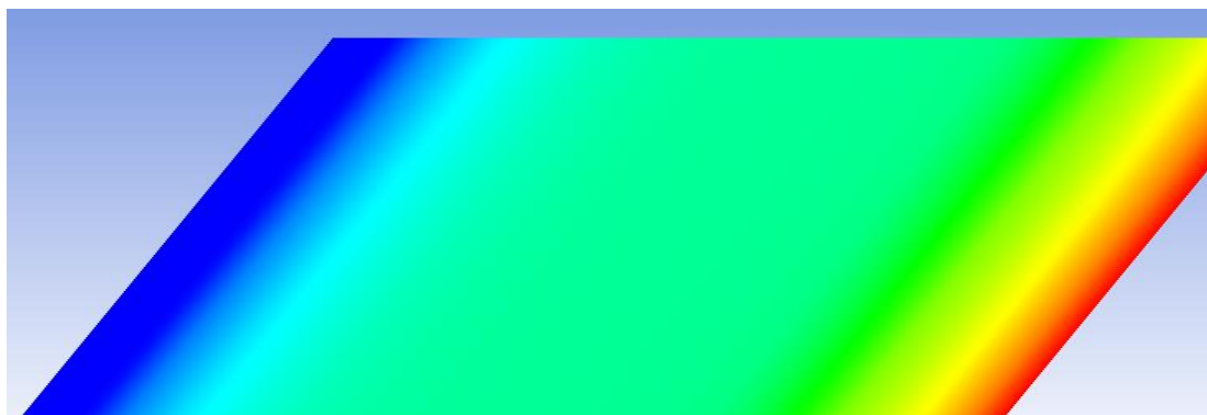
Slika 7.38 Polje temperature Ha < 1
