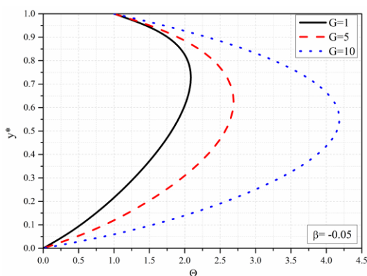
Slika 3.41b Bezdimeziona temperatura za različite vrednosti G , \beta = -0.05
