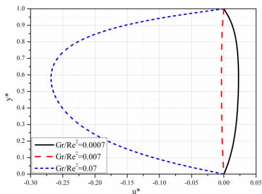
Slika 5.7 Bezdimezijska uzdužna brzina za različite vrednosti Gr/Re^2
