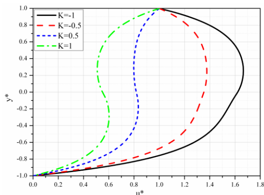
Slika 4.17 Bezdimezijska brzina za različite vrednosti K
