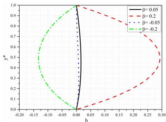
Slika 3.37 Bezdimeziona indukcija indukovanog magnetnog polja za razliĉite vrednosti \beta
