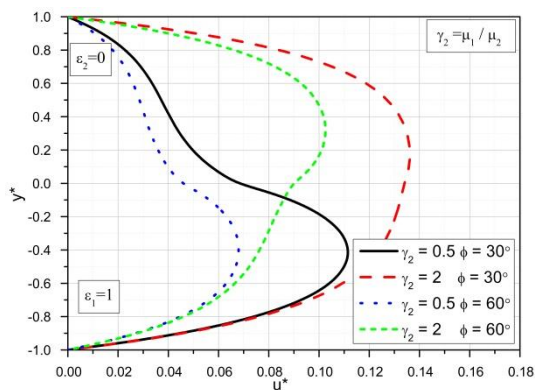
Slika 6.19 Bezdimezijska uzdužna brzina za različite vrednosti \gamma_2 i \phi
