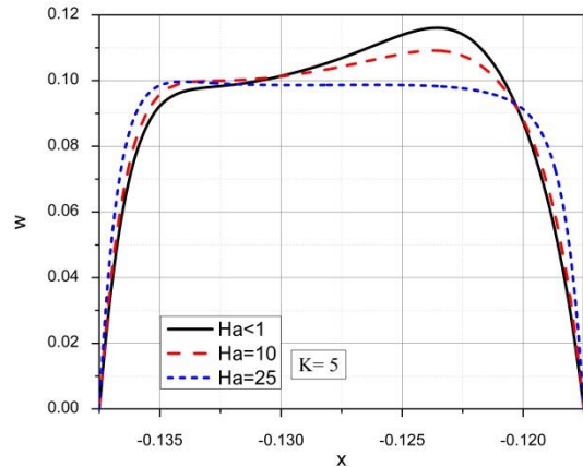
Slika 7.28 Uticaj Hartmann-ovog broja na komponentu brzine u z pravcu
