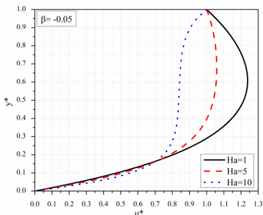
Slika 3.30b Bezdimezijska uzduzna brzina za različite vrednosti Ha , \beta = -0.05
