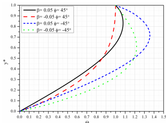
Slika 5.14 Bezdimezionna temperatura za različite vrednosti \phi i \beta
