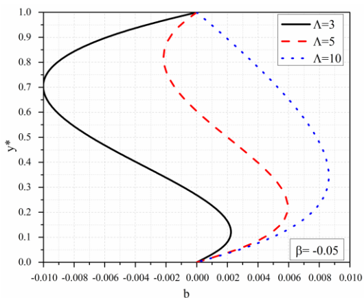
Slika 3.34b Bezdimezijska indukcija indukovano magnetnog polja za različite vrednosti \Lambda , \beta = -0.05
