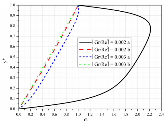
Slika 5.49 Bezdimezijska temperatura za različite vrednosti Gr/Re^2
