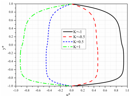
Slika 4.5 Bezdimezijska brzina za različite vrednosti K
