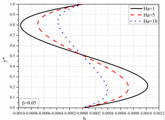
Slika 3.22 Bezdimeziona indukcija indukovanog magnetnog polja za različite vrednosti Ha
