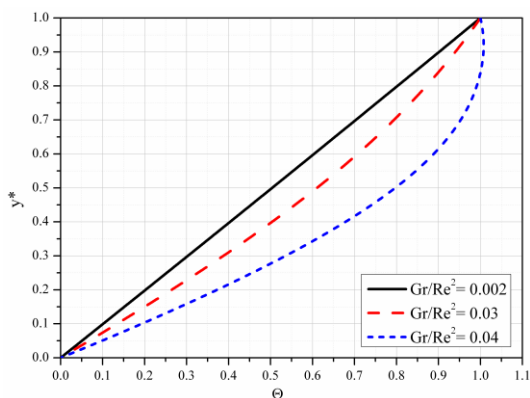
Slika 5.8 Bezdimezijska temperatura za različite vrednosti Gr/Re^2
