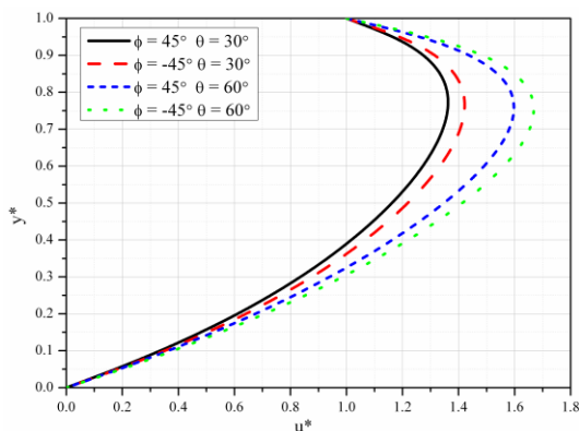
Slika 5.31 Bezdimezijska uzdužna brzina za različite vrednosti \phi i \theta
