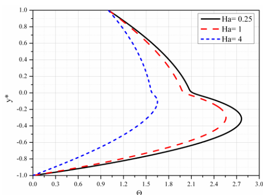
Slika 4.22 Bezdimezionizovana temperatura za različite vrednosti odnosa Hartmann-ovih brojeva Ha
