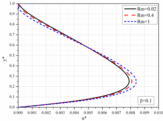
Slika 3.46a Bezdimezijska uzdužna brzina za različite vrednosti R_m , \beta = 0.1, c = 1, Ha = 10
