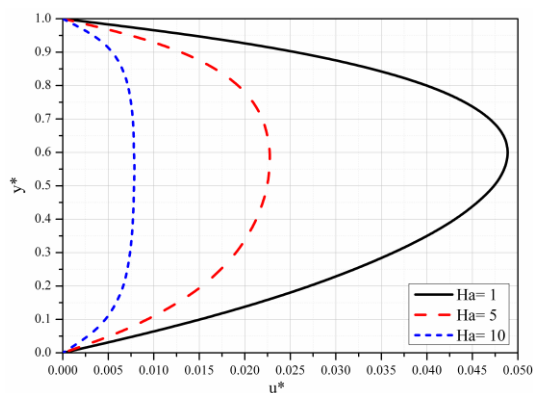
Slika 5.1 Rasplet bezdimenzionirane uzdužne brzine za različite vrednosti Hartmann-ovog broja
