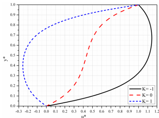
Slika 5.23 Bezdimezijska uzdužna brzina za različite vrednosti K
