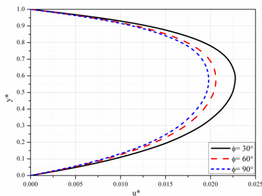
Slika 5.9 Bezdimezijska uzdužna brzina za različite vrednosti \phi
