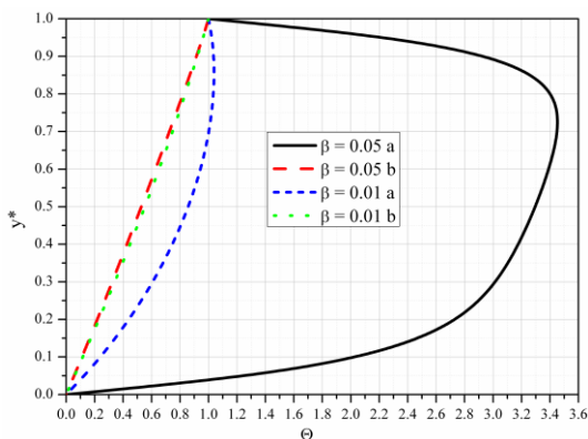
Slika 5.46 Bezdimezijska temperatura za različite vrednosti \beta
