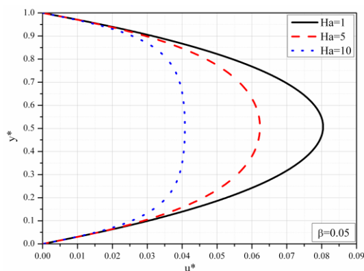
Slika 3.17 Bezdimezionna uzdužna brzina za različite vrednosti Ha
