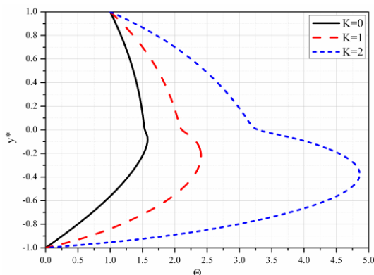
Slika 4.24 Bezdimenziona temperatura za različite vrednosti K
