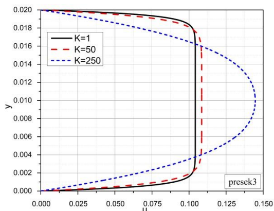
Slika 7.9 Bezdimezijska uzdužna brzina za različite vrednosti faktora otpora sredine
