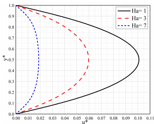
Slika 3.1 Raspoored uzdužne brzine za različite vrednosti Hartmann-ovog broja
