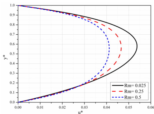
Slika 5.41 Bezdimeziona uzdužna brzina za različite vrednosti Rm
