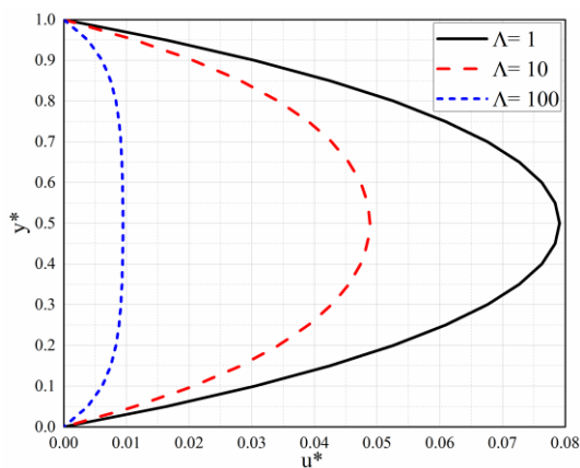
Slika 3.3 Raspored bezdimenzionirane brzine za različite vrednosti faktora poroznosti
