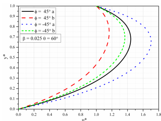
Slika 5.77 Bezdimezijska brzina za različite vrednosti \phi
