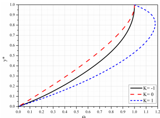
Slika 5.24 Bezdimezijska temperatura za različite vrednosti K
