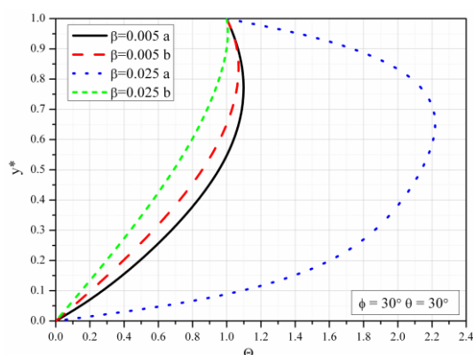
Slika 5.73 Bezdimezionna temperatura za različite vrednosti \beta , \phi = 30^\circ , \theta = 30^\circ
