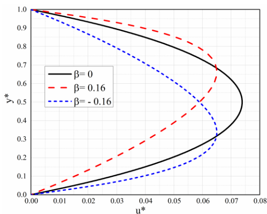
Slika 3.2 Raspoored bezdimenzionu uzdužne brzine za različite vrednosti faktora \beta
