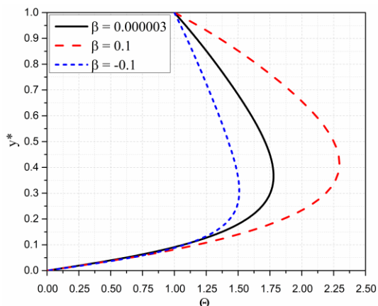
Slika 3.14 Raspored bezdimenzionih temperature za različite vrednosti \beta
