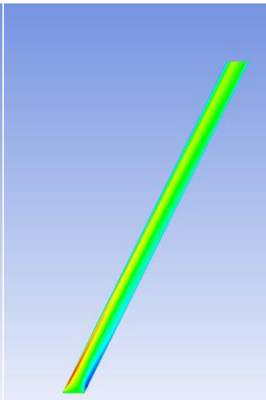
Slika 7.32 Komponenta brzine w u kosom kanalu
