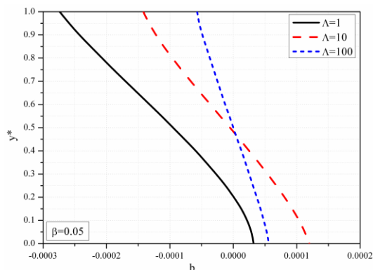
Slika 3.48a Bezdimeziona indukcija za različite vrednosti \Lambda , \beta = 0.05 , c = 1
