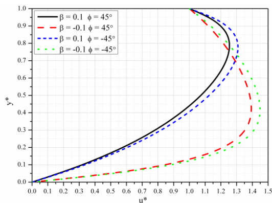
Slika 5.29 Bezdimezijska uzdužna brzina za različite vrednosti \beta i \phi
