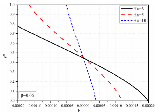
Slika 3.47a Bezdimezijska indukcija za različite vrednosti Ha, \beta = 0.05, c = 1 ,
