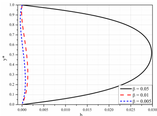
Slika 5.45 Bezdimezijska magnetna indukcija za različite vrednosti \beta
