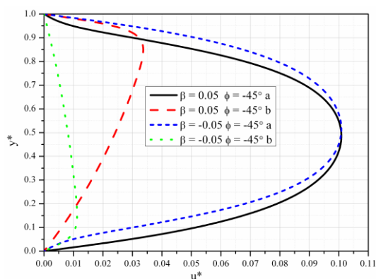
Slika 5.51 Bezdimeziono uzdužna brzina za različite vrednosti \beta i \phi = -45^\circ
