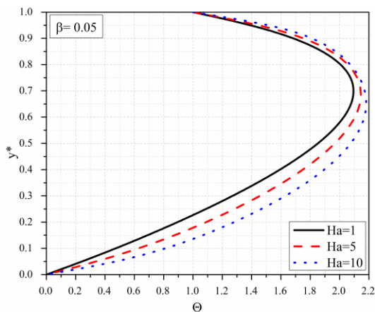
Slika 3.40a Bezdimeziona temperatura za različite vrednosti Ha , \beta = 0.05
