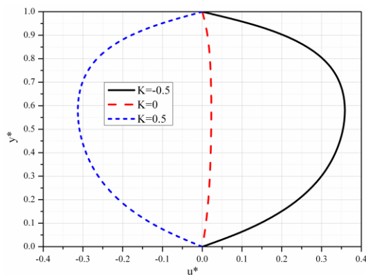
Slika 5.5 Bezdimezijska uzdužna brzina za različite vrednosti K
