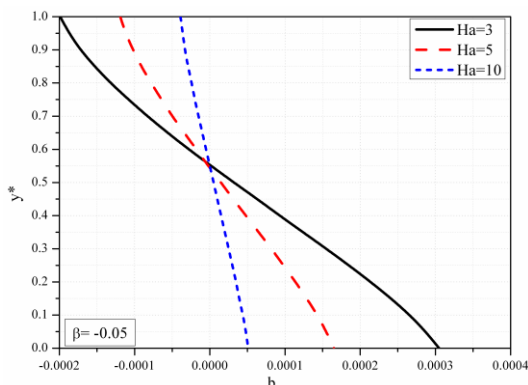
Slika 3.47b Bezdimezijska indukcija za različite vrednosti Ha, \beta = -0.05, c = 1
