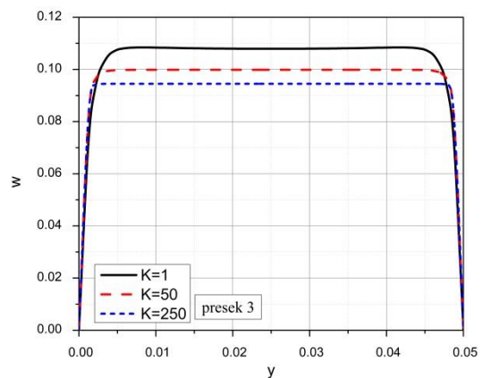
Slika 7.26 Uticaj faktora otpora sredine na komponentu brzine u z pravcu
