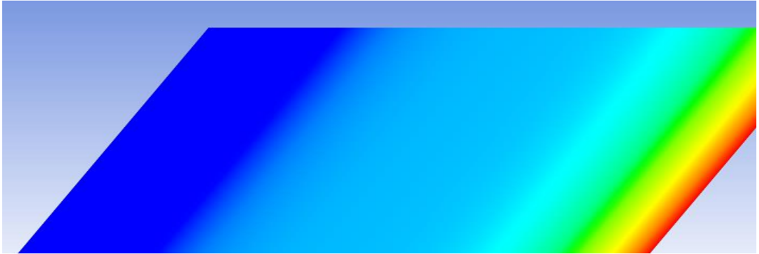
Slika 7.39 Polje temperature Ha=10
