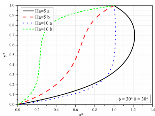
Slika 5.66 Bezdimenziona uzdužna brzina za različite vrednosti Ha broja, \phi = 30^\circ , \theta = 30^\circ
