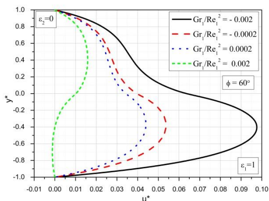
Slika 6.24 Bezdimezionna brzina za različite vrednosti Gr_1/Re_1^2 i \phi = 60^\circ
