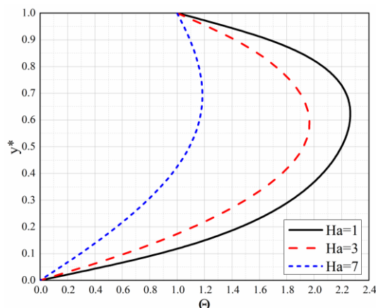
Slika 3.5 Rasporid bezdimenzionih temperature za različite vrednosti Hartmann-ovog broja
