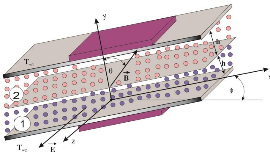
Slika 6a Fizički model strujanja
