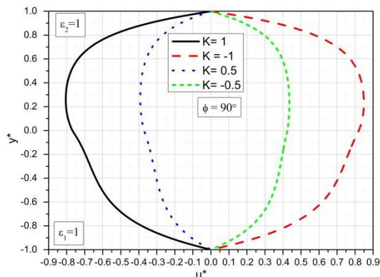
Slika 6.9 Bezdimezijska uzdužna brzina za različite vrednosti K i \phi = 90^\circ
