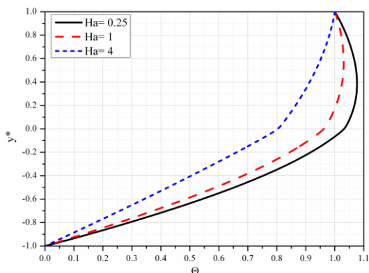
Slika 4.10 Bezdimezijska temperatura za različite vrednosti parametra Ha
