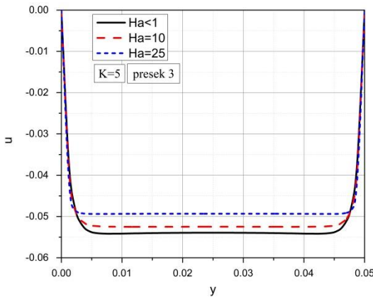
Slika 7.29 Uticaj Hartmann-ovog broja na komponentu brzine u x pravcu
