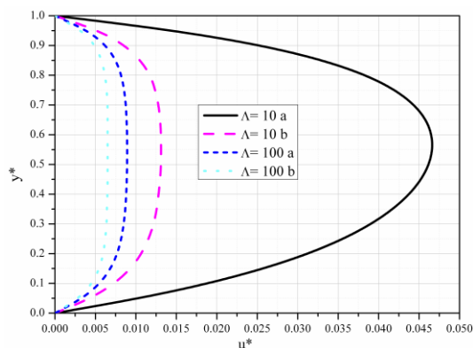
Slika 5.38 Bezdimezijska uzdužna brzina za različite vrednosti \Lambda
