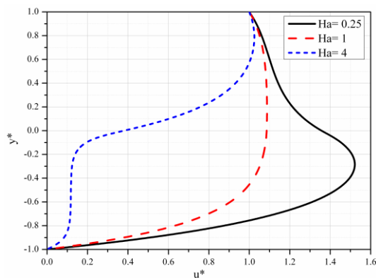
Slika 4.15 Bezdimezijska brzina za različite vrednosti odnosa Hartmann-ovih brojeva
