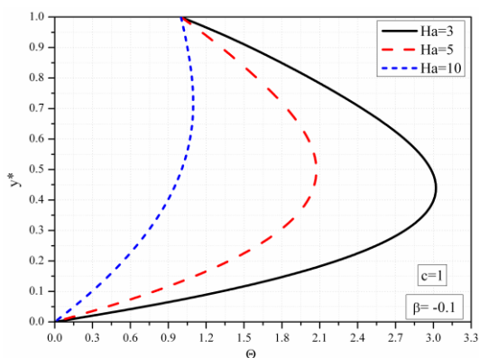
Slika 3.50b Bezdimezionna temperatura za različite vrednosti Ha , \beta = -0.1
