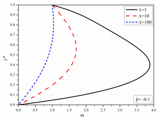
Slika 3.51b Bezdimezijska temperatura za različite vrednosti \Lambda, \beta = -0.1, c = 1
