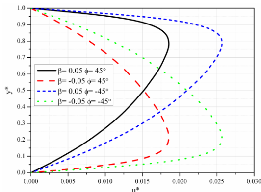
Slika 5.13 Bezdimezionna uzdužna brzina za različite vrednosti \phi i \beta
