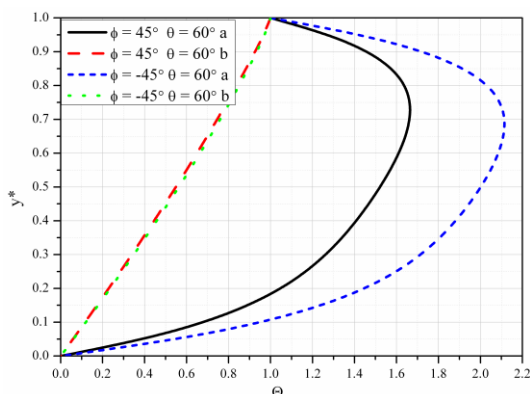
Slika 5.59 Bezdimezionna temperatura za različite vrednosti \phi i \theta = 60^\circ
