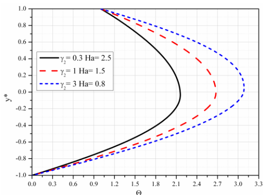
Slika 4.8 Bezdimezijska temperatura za različite vrednosti odnosa viskoznosti \gamma_2
