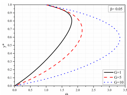
Slika 3.41a Bezdimeziona temperatura za različite vrednosti G , \beta = 0.05
