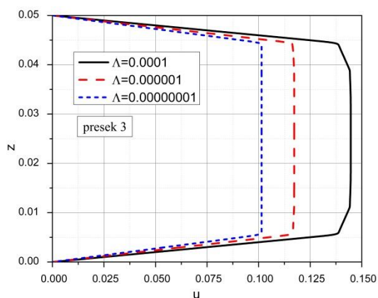
Slika 7.7 Bezdimezionna brzina za različite vrednosti poroznosti
