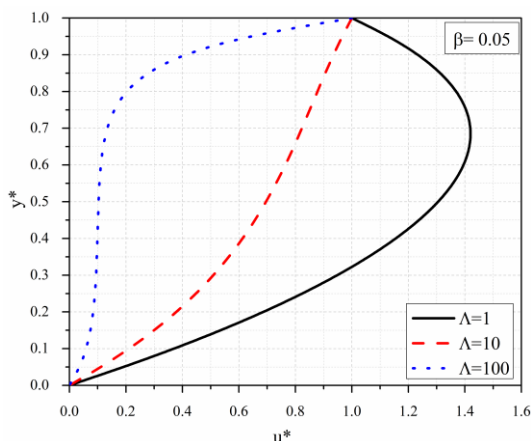
Slika 3.29a Bezdimeziorna uzdužna brzina za različite vrednosti \Lambda ; \beta = 0.05
