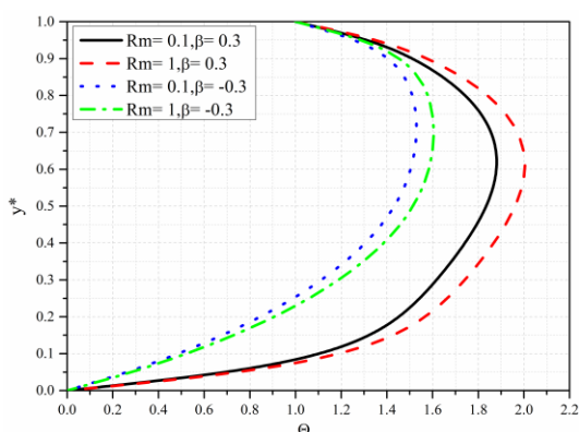
Slika 3.43 Bezdimezionna temperatura za različite vrednosti Rm i \beta
