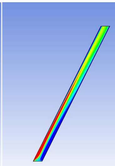
Slika 7.36 Polje brzine Ha = 10
