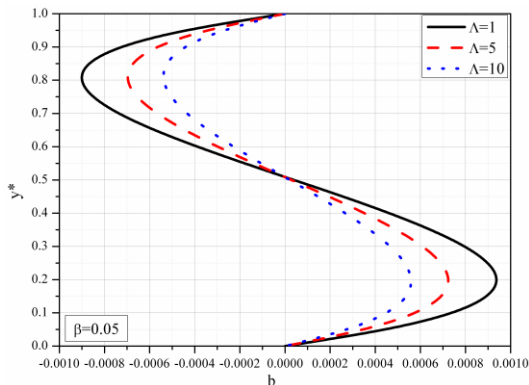
Slika 3.21 Bezdimeziona indukcija indukovanog magnetnog polja za različite vrednosti \Lambda
