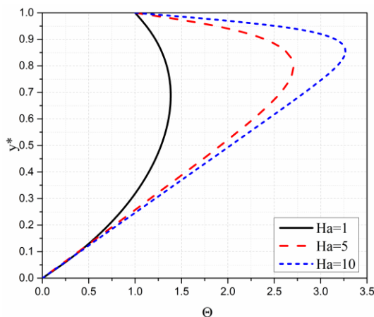
Slika 3.13 Raspored bezdimenzionih temperature za različite vrednosti Ha
