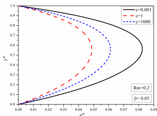
Slika 3.53 Bezdimeziona uzdužna brzina za različite vrednosti c , \beta = 0.05
