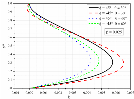
Slika 5.79 Bezdimeziono indukovano polje za različite vrednosti \phi
