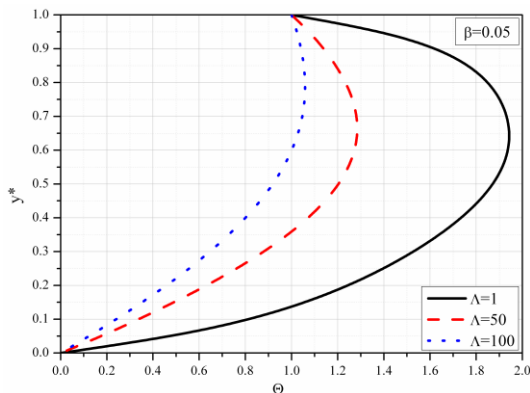
Slika 3.26 Bezdimezijska temperatura za različite vrednosti \Lambda
