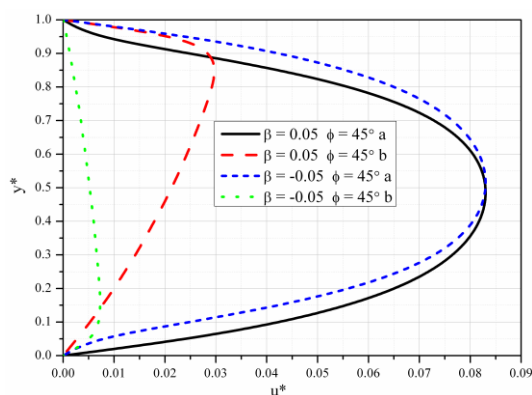
Slika 5.50 Bezdimeziono uzdužna brzina za različite vrednosti \beta i \phi = 45^\circ
