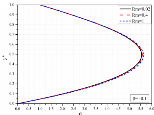
Slika 3.52b Bezdimezijska temperatura za različite vrednosti Rm , \beta = -0.1 , c = 1
