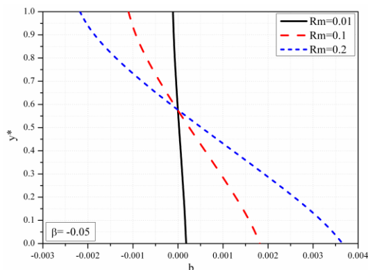
Slika 3.49b Bezdimezijska indukcija za različite vrednosti R_m , \beta = -0.05 , c = 1
