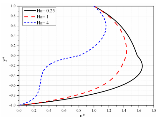
Slika 4.21 Bezdimezionizovana brzina za različite vrednosti odnosa Hartmann-ovih brojeva Ha
