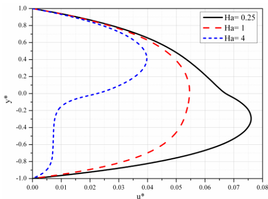
Slika 4.9 Bezdimezijska brzina za različite vrednosti parametra Ha
