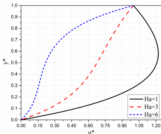
Slika 3.9 Raspored bezdimenzione brzine za različite vrednosti Ha
