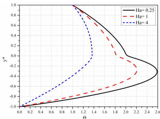
Slika 4.16 Bezdimezijska temperatura za različite vrednosti odnosa Hartmann-ovih brojeva
