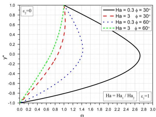
Slika 6.16 Bezdimezijska temperatura za različite vrednosti Ha i \phi
