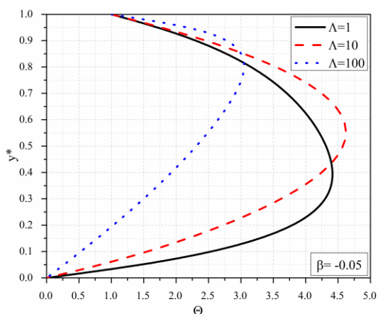
Slika 3.39b Bezdimeziona temperatura za različite vrednosti \Lambda , \beta = -0.05
