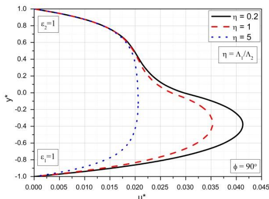
Slika 6.7 Bezdimezijska uzdužna brzina za različite vrednosti \eta i \phi = 90^\circ
