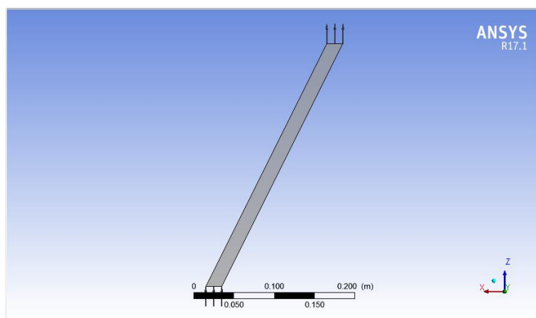
Slika 7.18. Model kosog kanala u ICEM-CFD-u
