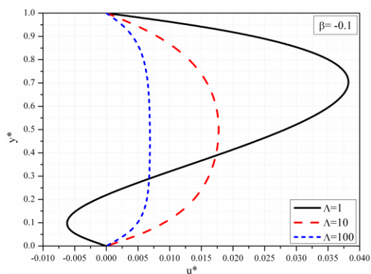
Slika 3.45b Bezdimeziono uzdužna brzina za različite vrednosti \Lambda , \beta = -0.1 , c = 1
