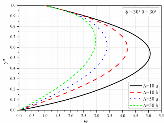
Slika 5.70 Bezdimeziona temperatura za različite vrednosti \Lambda , \phi = 30^\circ , \theta = 30^\circ
