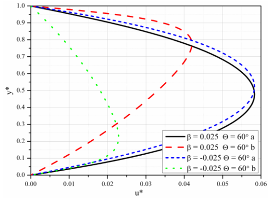
Slika 5.61 Bezdimezijska uzdužna brzina za različite vrednosti \beta i \theta = 60^\circ
