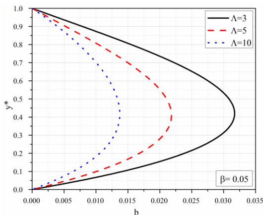
Slika 3.34a Bezdimezijska indukcija indukovano magnetnog polja za različite vrednosti \Lambda , \beta = 0.05
