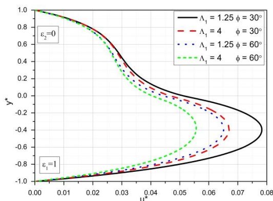
Slika 6.11 Bezdimeziorna uzdužna brzina za različite vrednosti \Lambda_1 i \phi
