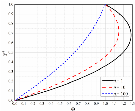
Slika 3.7 Rasped bezdimenzionane temperature za različite vrednosti faktora poroznosti
