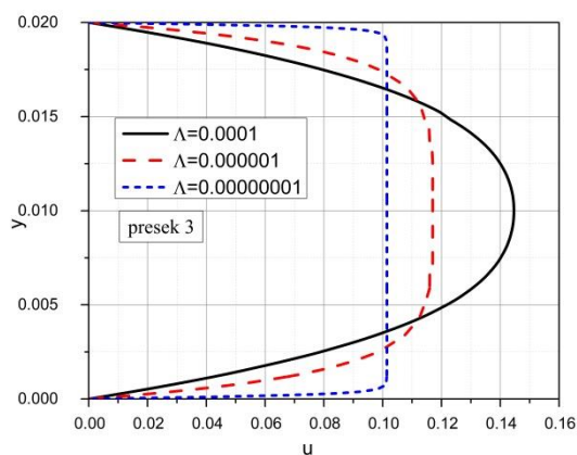
Slika 7.6 Bezdimezionna uzdužna brzina za različite vrednosti poroznosti
