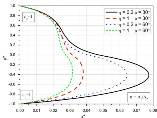
Slika 6.1 Bezdimezionna uzdužna brzina za različite vrednosti \eta i \phi
