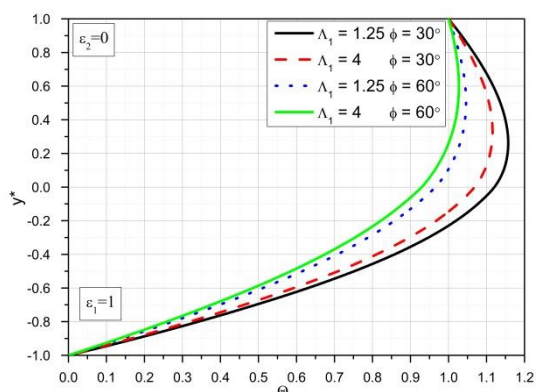
Slika 6.12 Bezdimeziorna temperatura za različite vrednosti \Lambda_1 i \phi
