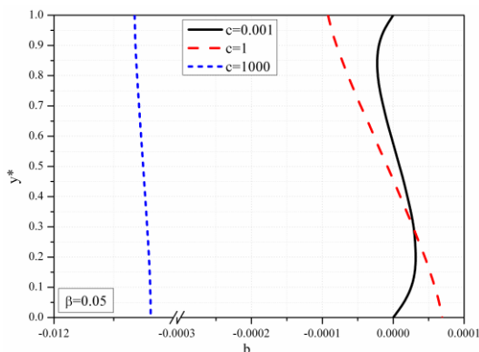
Slika 3.55 Bezdimeziiona magnetna indukcija za različite vrednosti c , \beta = 0.05
