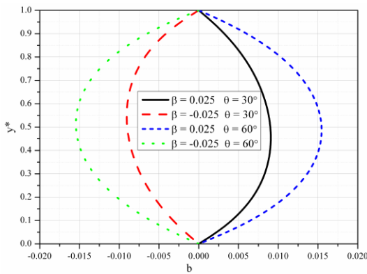
Slika 5.62 Bezdimezijska magnetna indukcija za različite vrednosti \beta i \theta
