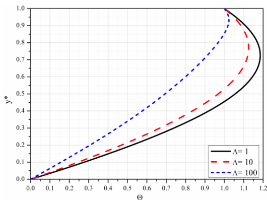
Slika 5.22 Bezdimezijska temperatura za različite vrednosti \Lambda
