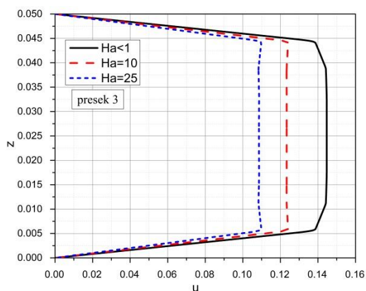
Slika 7.12 Bezdimezijska uzdužna brzina za različite vrednosti Hartmann-ovog broja
