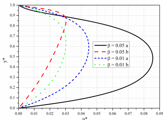
Slika 5.44 Bezdimezijska uzdužna brzina za različite vrednosti \beta
