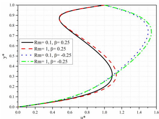
Slika 3.33 Bezdimezijska uzdužna brzina za različite vrednosti Rm i \beta
