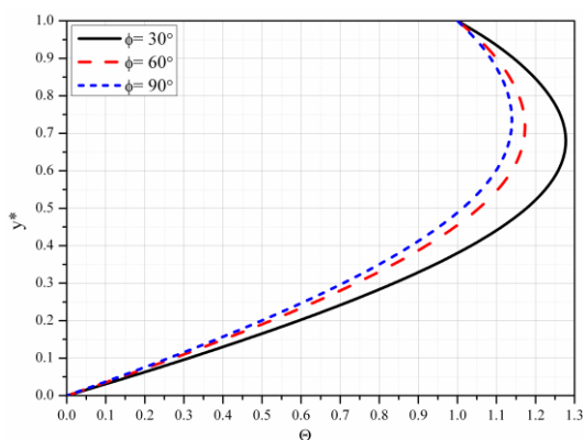
Slika 5.10 Bezdimezijska temperatura za različite vrednosti \phi
