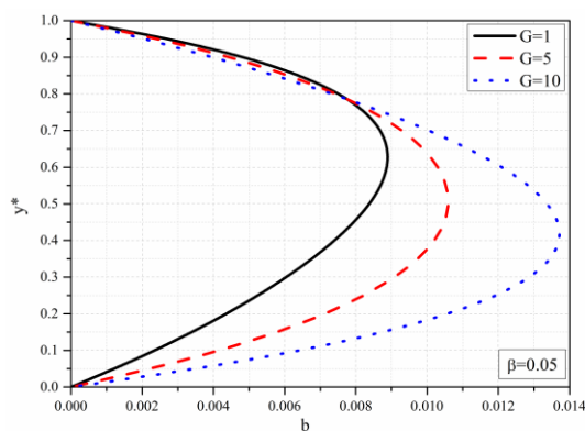
Slika 3.36a Bezdimeziona indukcija indukovanog magnetnog polja za razliĉite vrednosti G , \beta = 0.05
