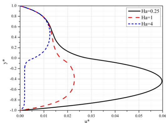
Slika 4.3 Bezdimezijska brzina za različite vrednosti Ha
