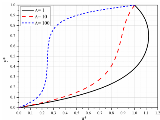
Slika 5.21 Bezdimezijska uzdužna brzina za različite vrednosti \Lambda
