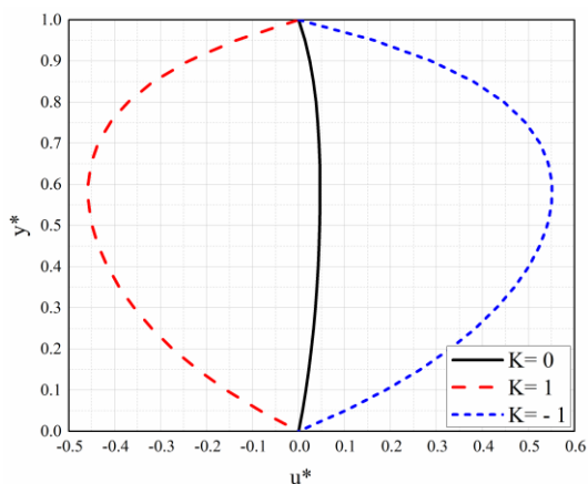
Slika 3.4 Raspored bezdimenzionirane brzine za različite vrednosti faktora električnega opterećenja
