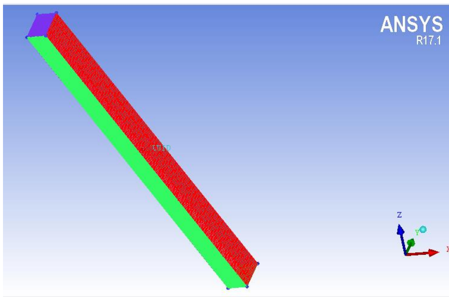
Slika 7.19. Domen strujanja u kosom kanalu
