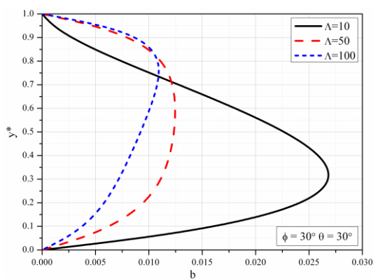
Slika 5.68 Bezdimezionno magnetno polje za različite vrednosti \Lambda , \phi = 30^\circ , \theta = 30^\circ
