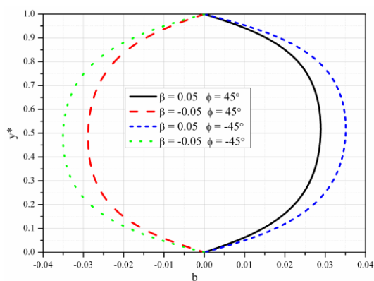
Slika 5.52 Bezdimeziono indukovan polje za različite vrednosti \beta i \phi
