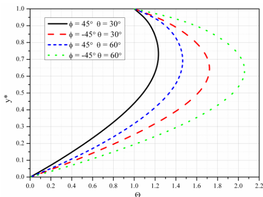
Slika 5.16 Bezdimezijska temperatura za različite vrednosti \phi i \theta
