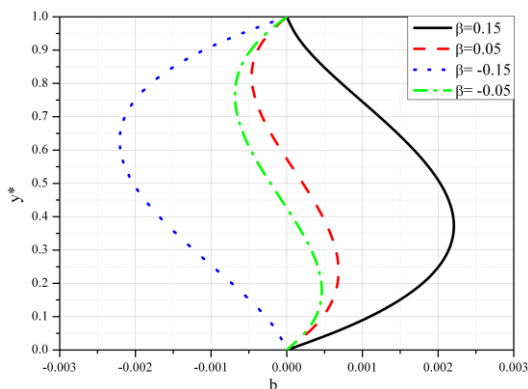
Slika 3.24 Bezdimezijska indukcija indukovano magnetnog polja za različite vrednosti \beta
