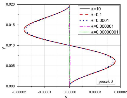
Slika 7.8 Bezdimeziona poprečna brzina za različite vrednosti poroznosti
