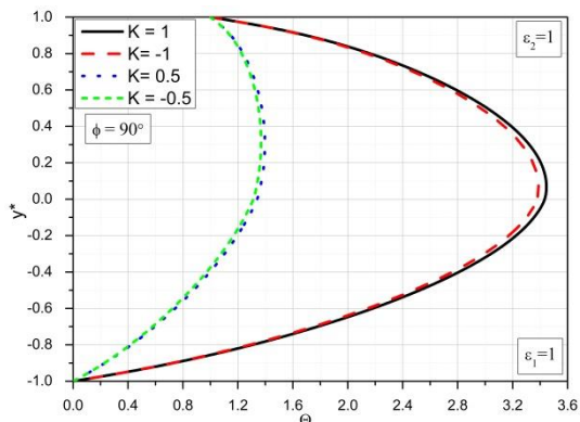
Slika 6.10 Bezdimezijska temperatura za različite vrednosti K i \phi = 90^\circ
