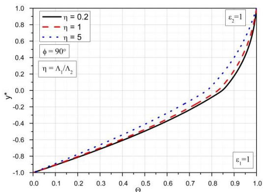
Slika 6.8 Bezdimezijska temperatura za različite vrednosti \eta i \phi = 90^\circ
