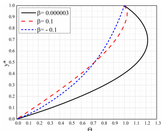
Slika 3.6 Rasporid bezdimenzionih temperature za različite vrednosti faktora \beta
