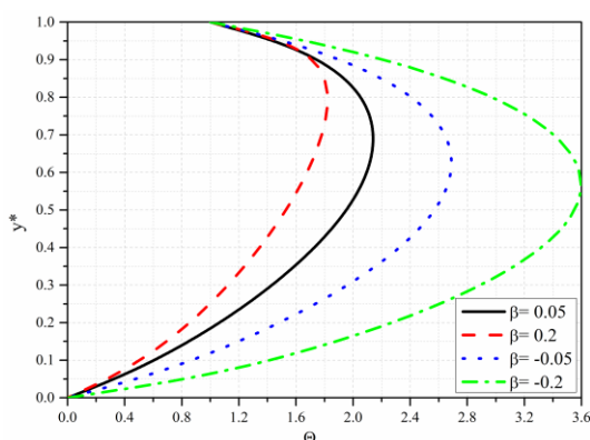
Slika 3.42 Bezdimezionna temperatura za različite vrednosti \beta
