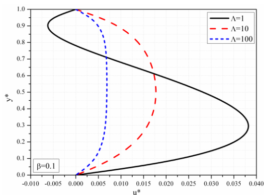
Slika 3.45a Bezdimeziono uzdužna brzina za različite vrednosti \Lambda , \beta = 0.1 , c = 1
