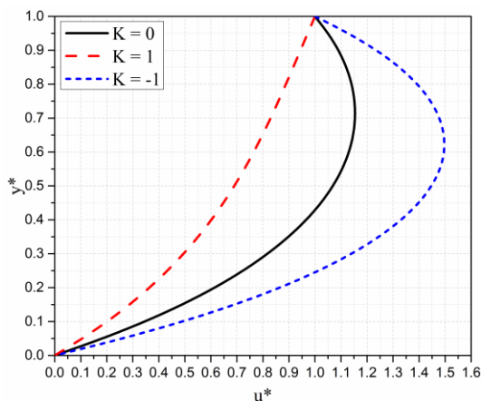
Slika 3.12 Raspojed bezdimenzionih brzina za različite vrijednosti K
