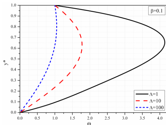
Slika 3.51a Bezdimezijska temperatura za različite vrednosti \Lambda, \beta = 0.1, c = 1
