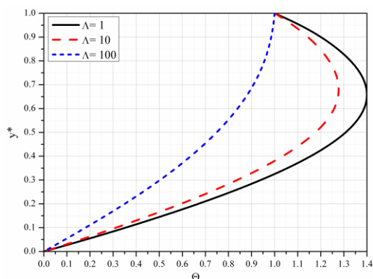
Slika 5.4 Raspored bezdimenzionirane temperature za različite vrednosti faktora poroznosti
