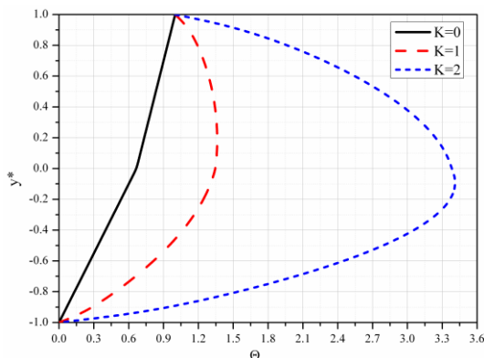
Slika 4.6 Bezdimezijska temperature za različite vrednosti K
